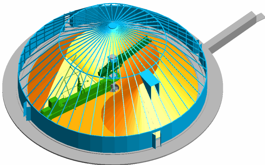
Трехмерные модели современного цементного завода и усреднительного склада
