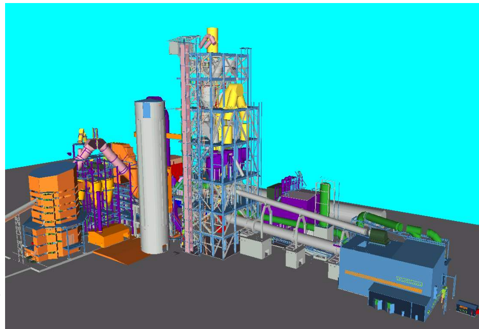
Трехмерные модели современного цементного завода и усреднительного склада
