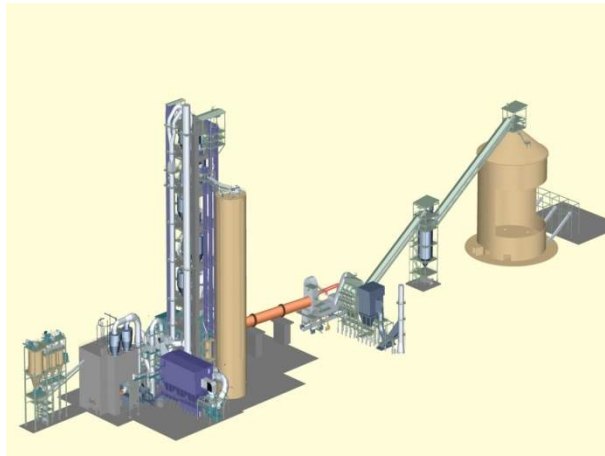
ОАО «Искитимцемент» общий вид новой линии
