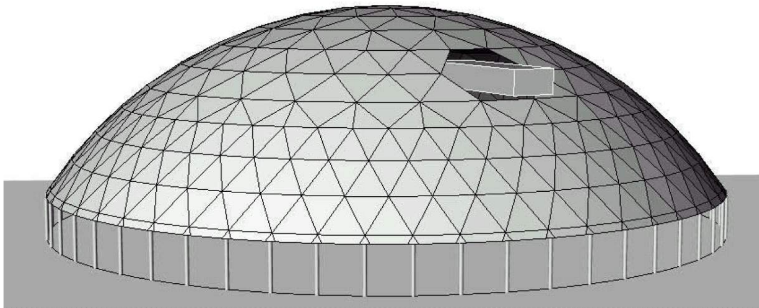
Расчетная модель купола шатрового склада диаметром 98 м
