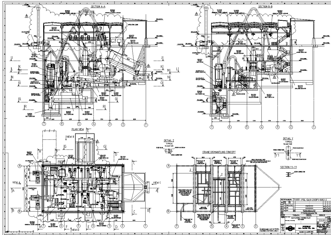
Примеры рабочих чертежей дробильного отделения известняка и глины из проекта цементного завода компании «PT Holcim Indonesia Tbk»
